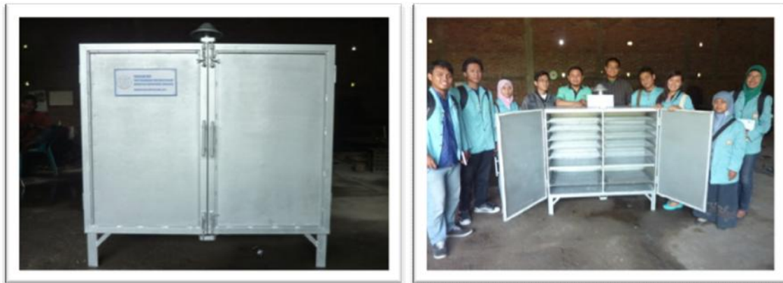
Gambar 1. Desain Alat Pengering-Tray Dryer Berbahan Bakar Biomassa
