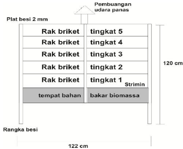
Gambar 1. Desain Alat Pengering-Tray Dryer Berbahan Bakar Biomassa
